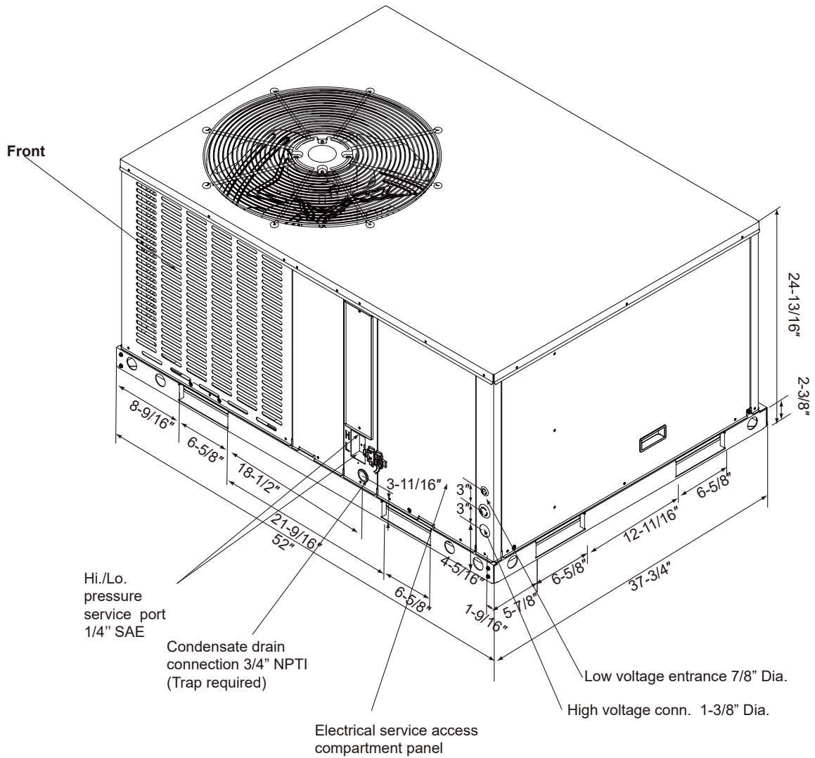
Fig. 2-2 Unit Dimensions
